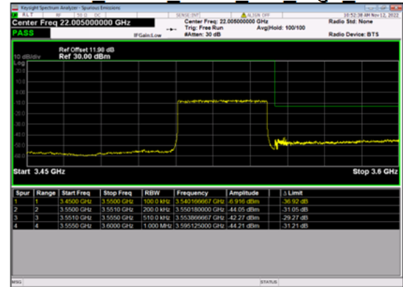
n77(60M)_DFT-s-OFDM QPSK Edge 1RB Left Low CH
