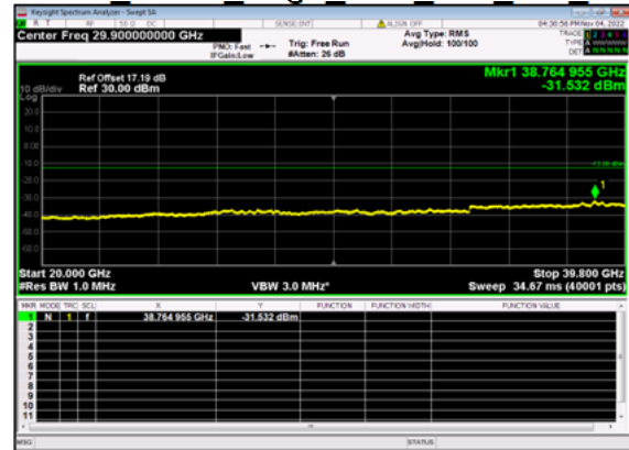
n77(20M)_DFT-s-OFDM BPSK Edge 1RB Left Mid CH
