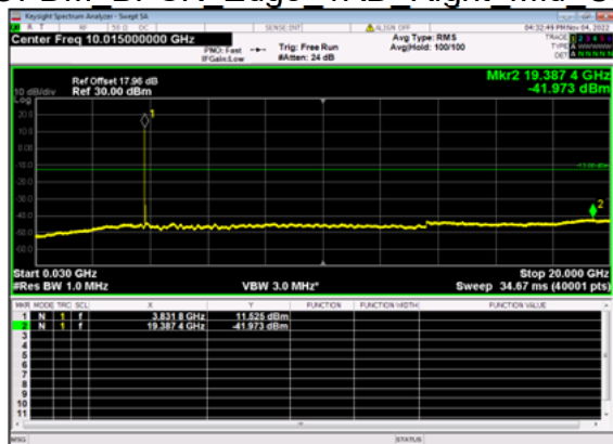
n77(20M)_DFT-s-OFDM BPSK Edge 1RB Right Mid CH
