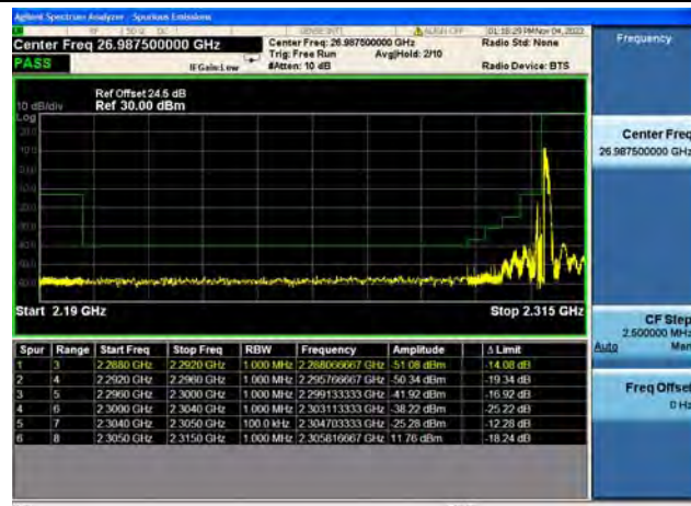
Band40 / 10MHz / Low CH / QPSK / 1 RB
