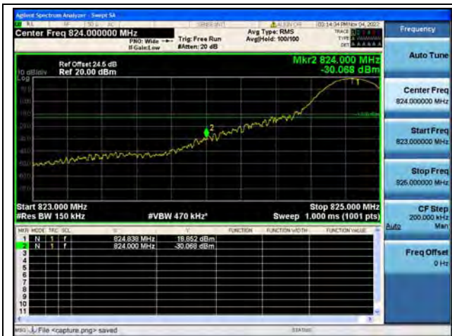
Band26 / 15MHz / Low CH / QPSK / 1 RB
