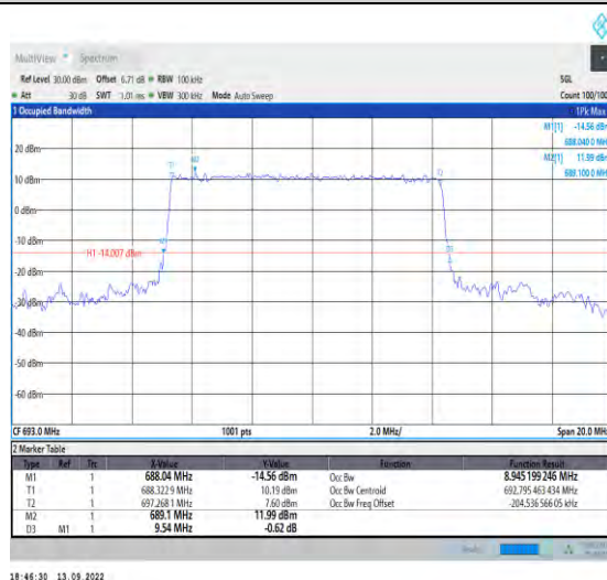
1-N71-15-10-H-3-DFT-16QAM-Outet_Full-50@0-Ant 1-8.945-9.540-≤10-PASS
