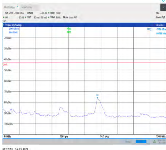
1-N66-PC3-15-40-H-1-DFT-PI2BPSK-Inner_1RB_L eft-1@1-0.009-0.15-Ant1-0.09--76.86--43-PASS
