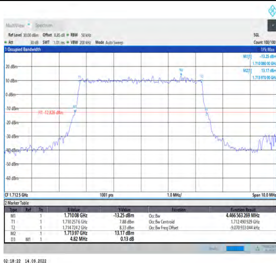
1-N66-PC3-15-5-L-3-DFT-16QAM-Outet_Full-25@0- Ant1-4.467-4.820-≤5-PASS
