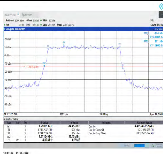
1-N66-PC3-15-5-L-4-DFT-64QAM-Outet_Full-25@0- Ant1-4.466-4.890-≤5-PASS
