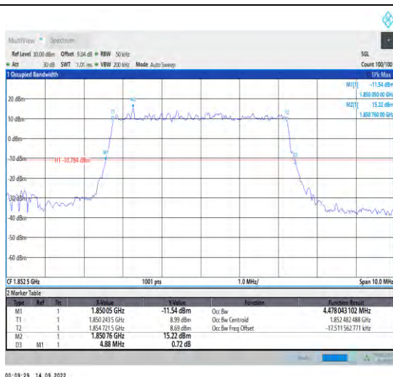
1-N25-PC3-15-5-L-1-DFT-QPSK-Outer_Full-25@0-A nt1-4.478-4.880-≤5-PASS
