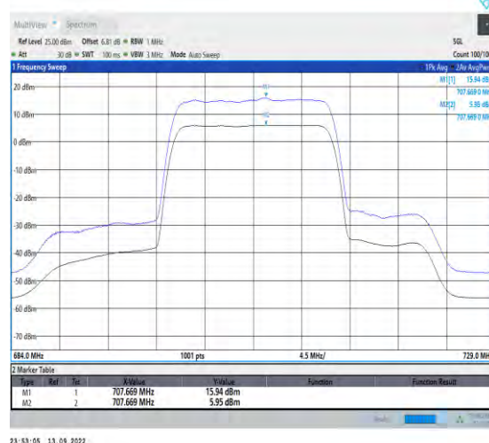
1-N12-PC3-15-15-L-2-CP-256QAM-Outer_Full-79@0 -Ant1-9.99-100%-0.00-9.99-PASS-≤13
