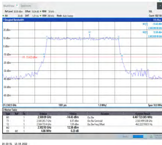
1-N7-PC3-15-5-L-3-DFT-16QAM-Outer_Full-25@0-A nt1-4.468-4.860-≤5-PASS
