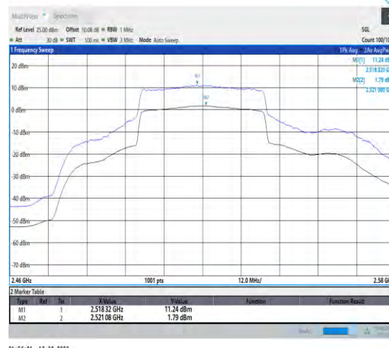
1-N7-PC3-15-40-L-2-CP-256QAM-Outet_Full-216@ 0-Ant1-9.45-100%-0.00-9.45-PASS-≤13
