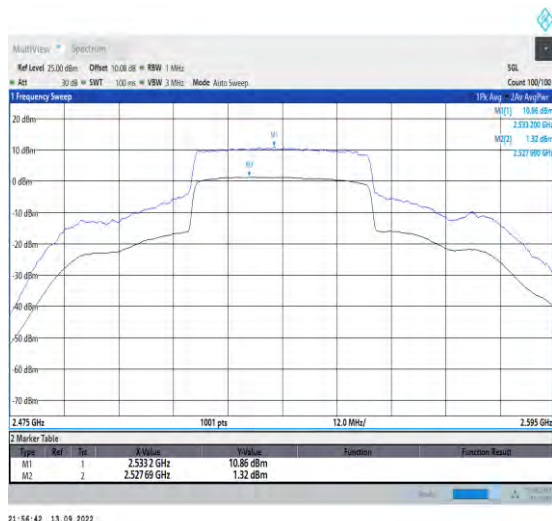
1-N7-PC3-15-40-M-1-DFT-256QAM-Outet_Full-216@ 0-Ant1-9.54-100%-0.00-9.54-PASS-≤13
