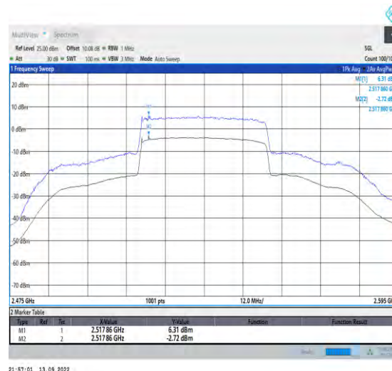
1-N7-PC3-15-40-M-2-CP-256QAM-Outet_Full-216@ 0-Ant1-9.03-100%-0.00-9.03-PASS-≤13
