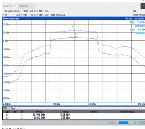
1-N7-PC3-15-40-L-1-DFT-256QAM-Outet_Full-216@ 0-Ant1-9.13-100%-0.00-9.13-PASS-≤13
