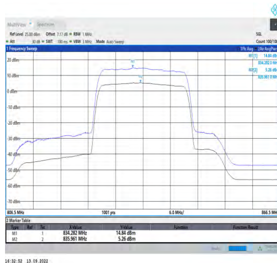
1-N5-PC3-15-20-M-2-CP-256QAM-Outer_Full-106@ 0-Ant1-9.58-100%-0.00-9.58-PASS-≤13
