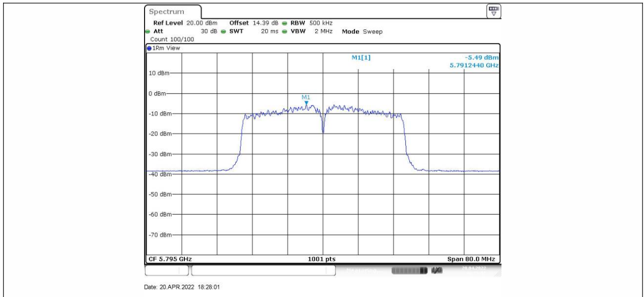
11N40SISO_Ant2_5795
