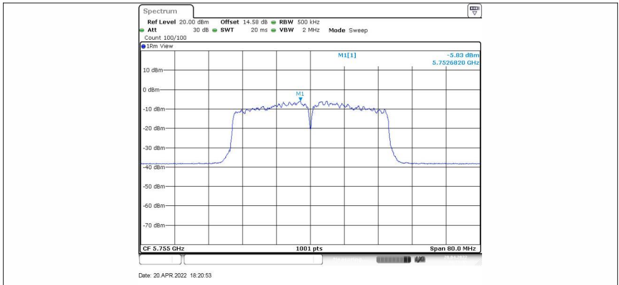
11N40SISO_Ant2_5755
