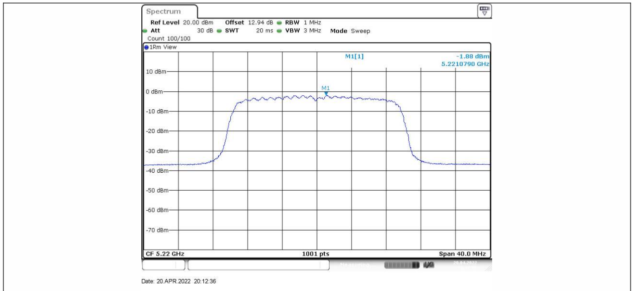
11AX20SISO_Ant2_5220
