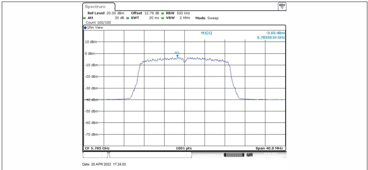
11N20SISO_Ant2_5785
