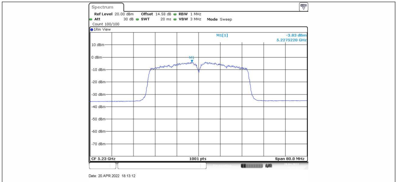
11N40SISO_Ant2_5230
