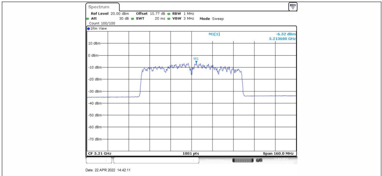
11AC80SISO_Ant2_5210
