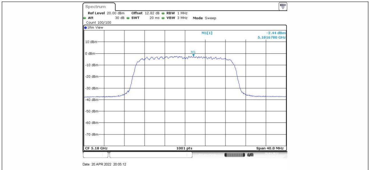
11AX20SISO_Ant2_5180
