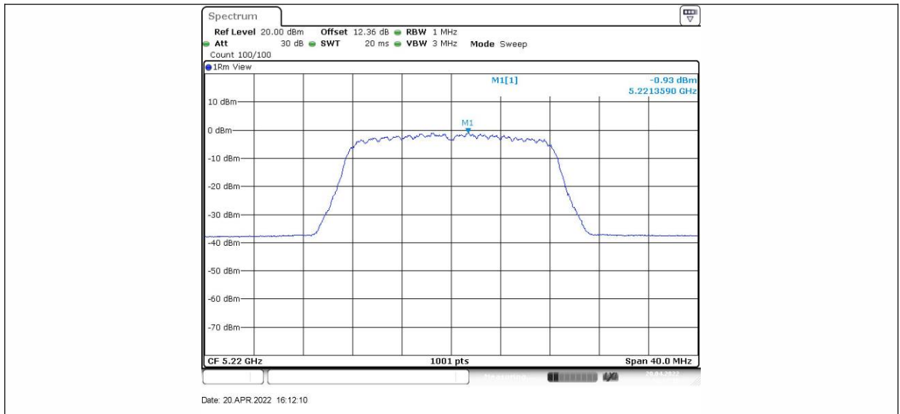
11A_Ant2_5220
