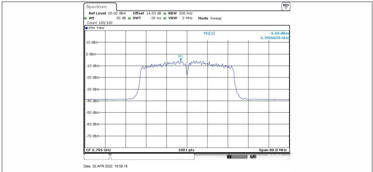
11AC40SISO_Ant2_5795
