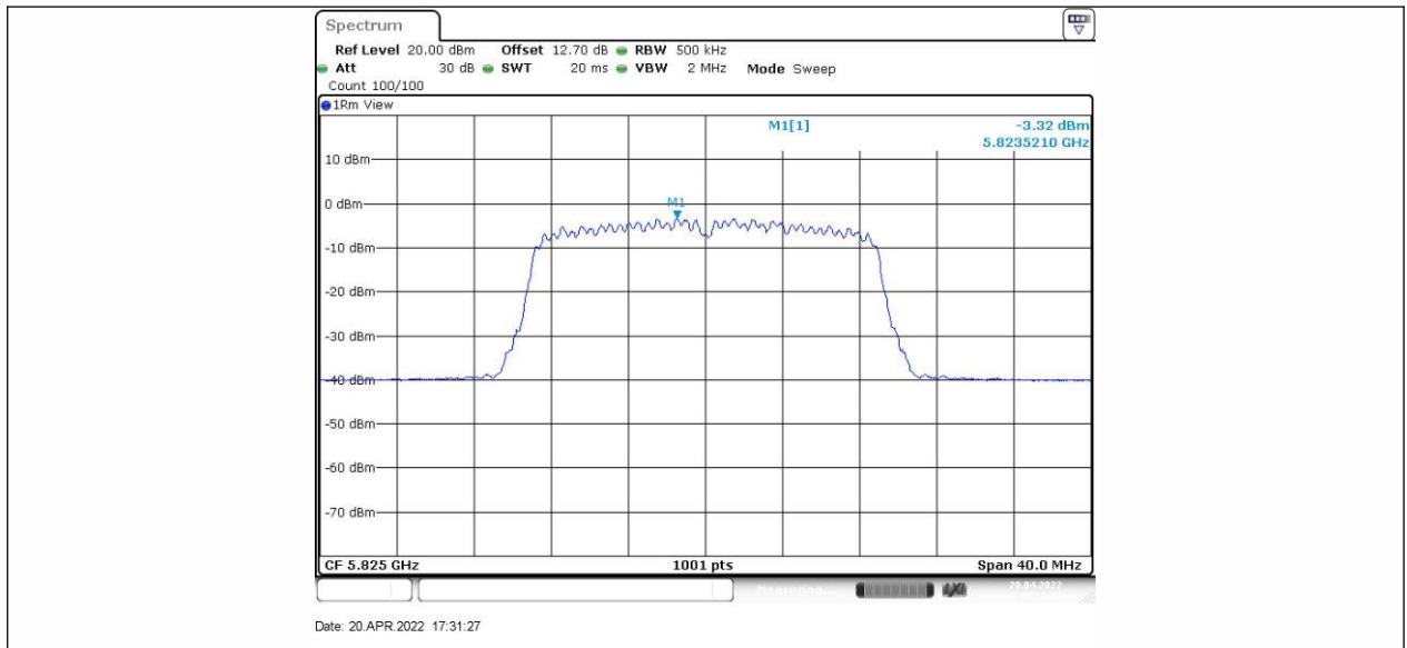
11N20SISO_Ant2_5825
