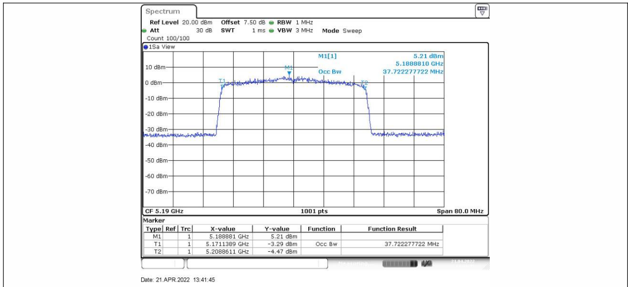
11AX40SISO_Ant2_5190
