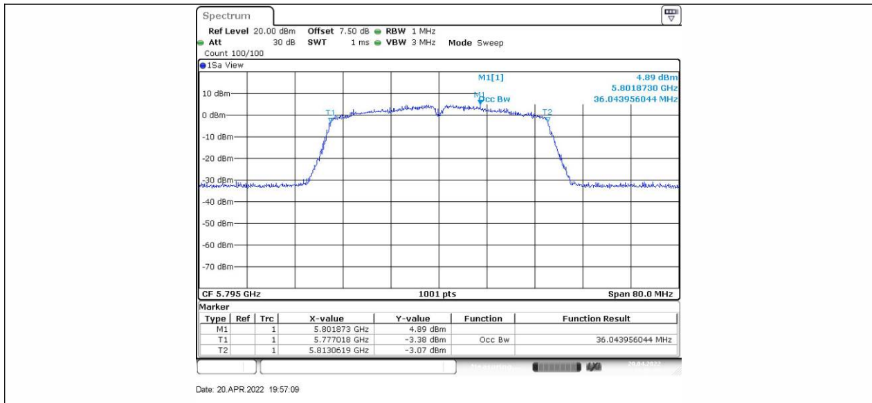
11AC40SISO_Ant2_5795
