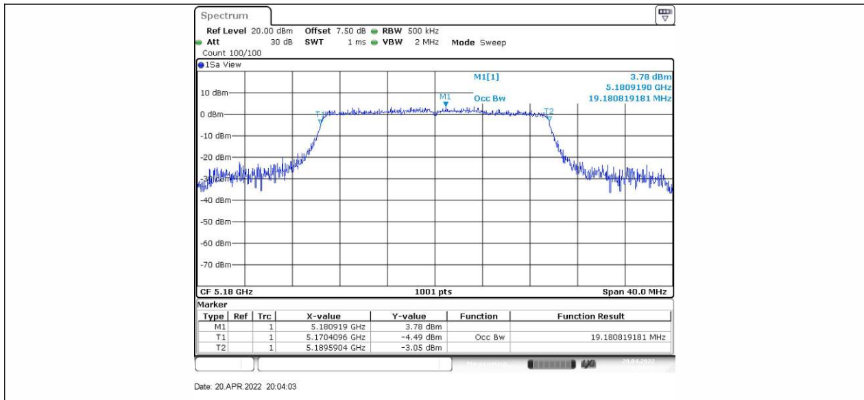
11AX20SISO_Ant2_5180
