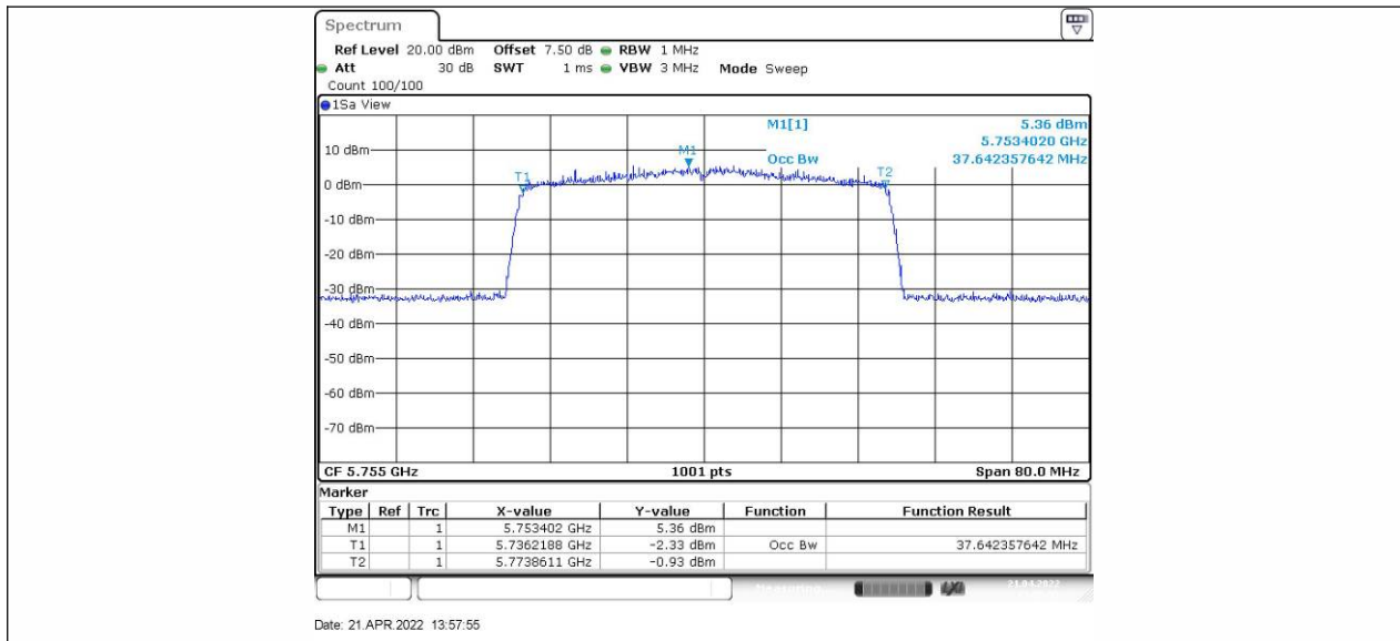
11AX40SISO_Ant2_5755
