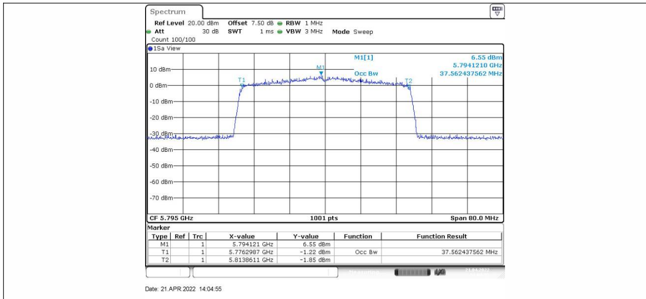
11AX40SISO_Ant2_5795
