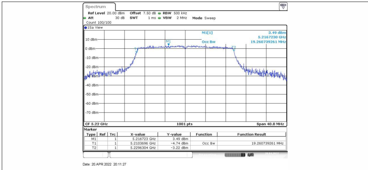
11AX20SISO_Ant2_5220
