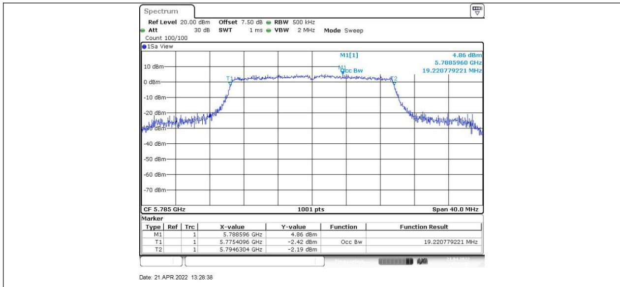
11AX20SISO_Ant2_5785
