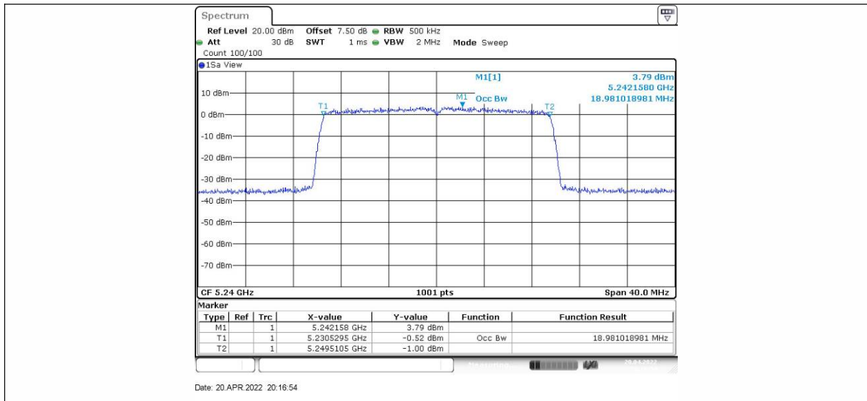
11AX20SISO_Ant2_5240
