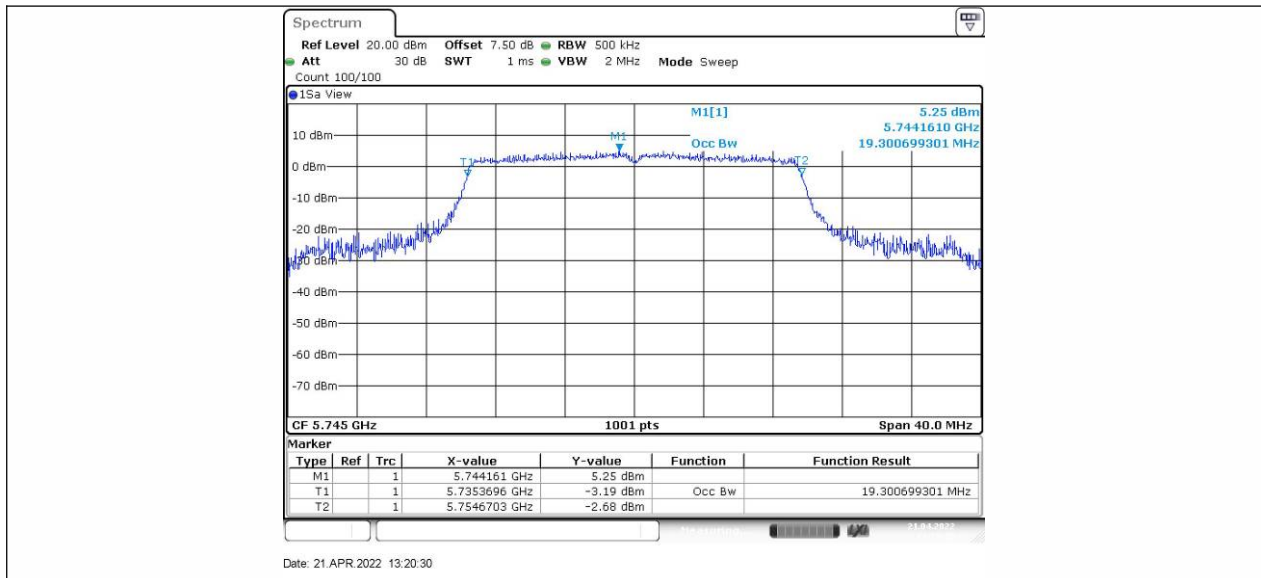
11AX20SISO_Ant2_5745
