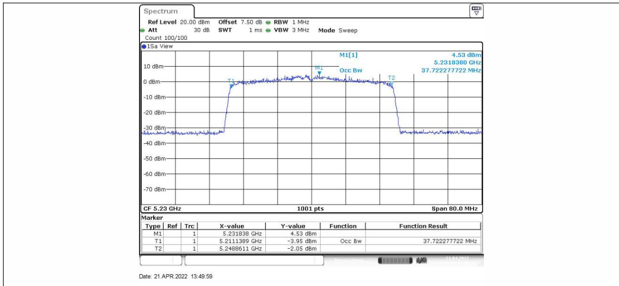
11AX40SISO_Ant2_5230
