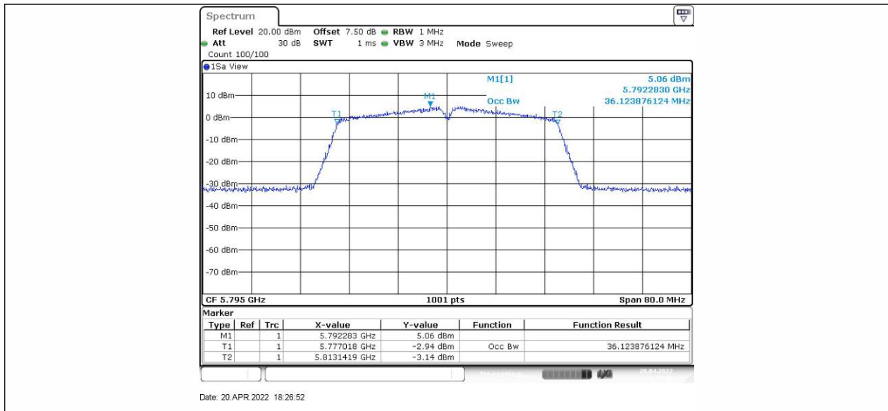
11N40SISO_Ant2_5795
