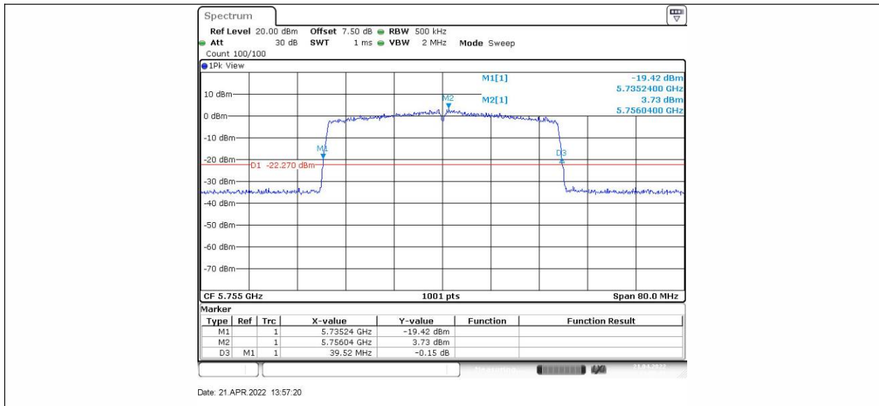
11AX40SISO_Ant2_5755
