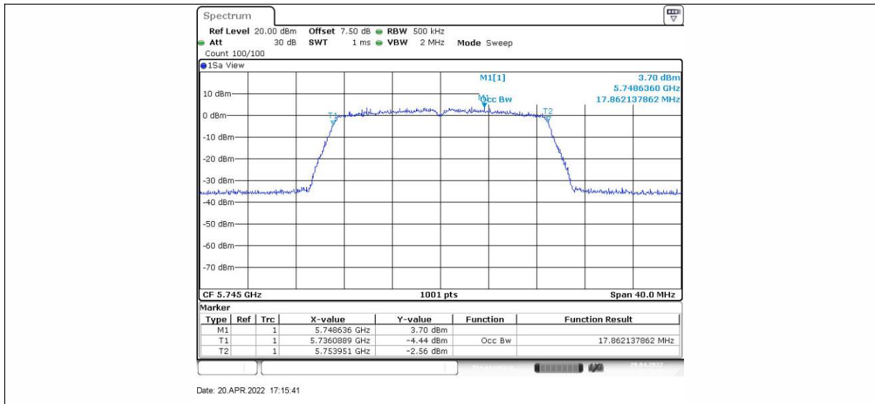
11N20SISO_Ant2_5745
