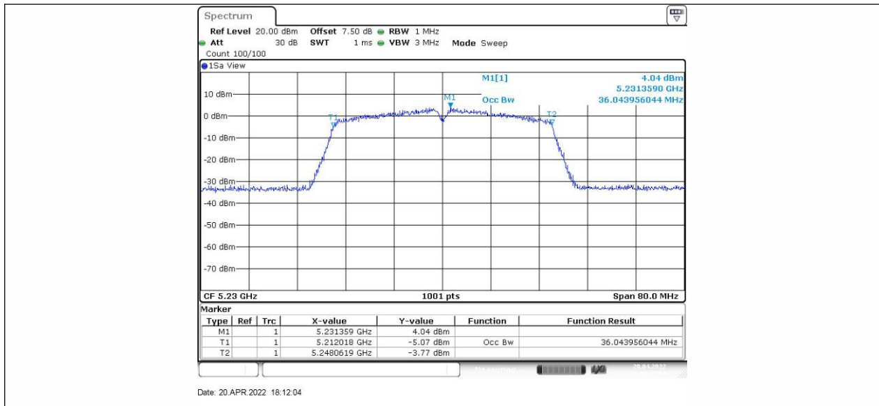
11N40SISO_Ant2_5230
