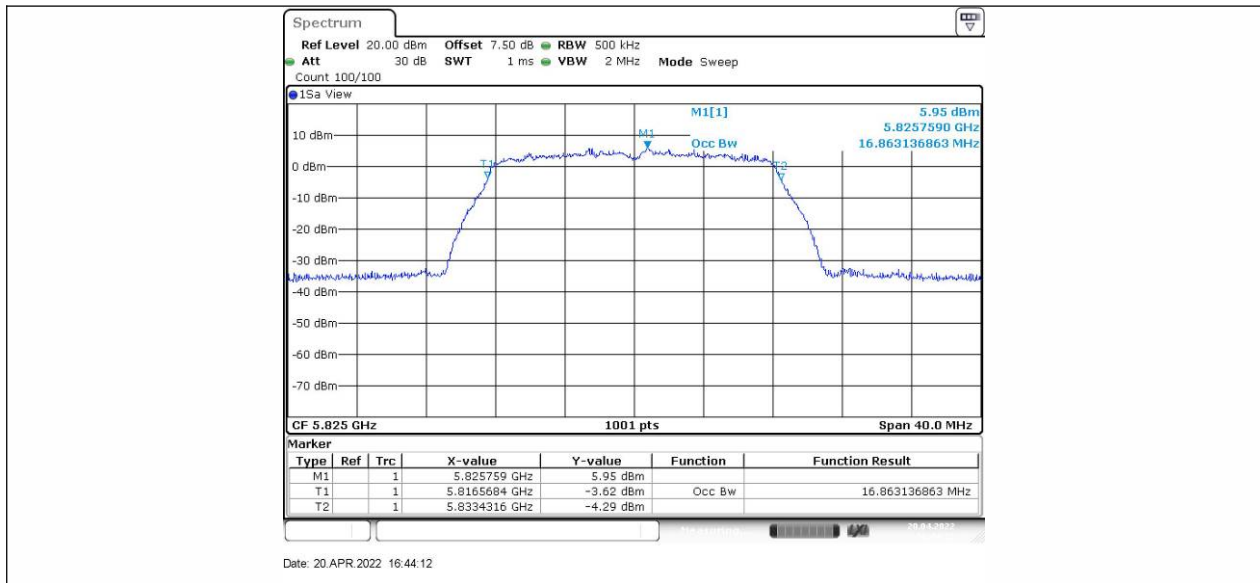
11A_Ant2_5825
