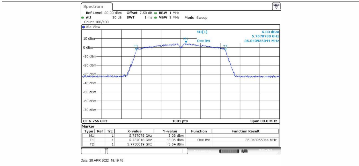
11N40SISO_Ant2_5755
