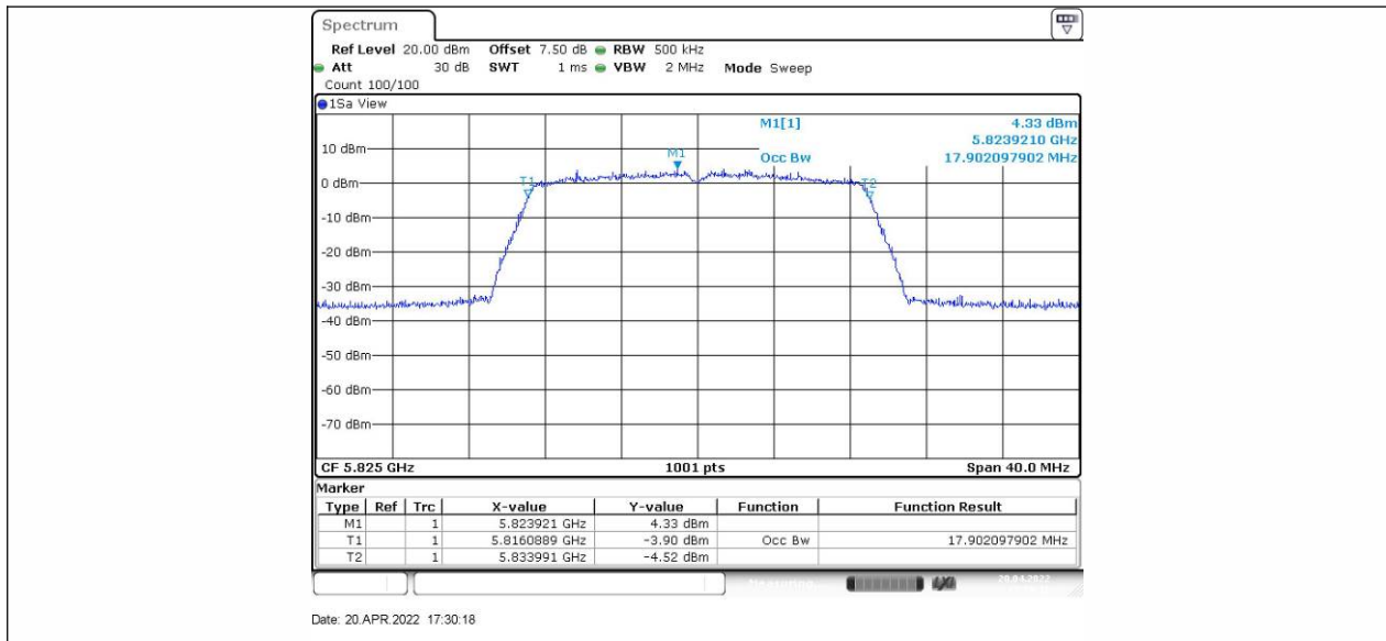
11N20SISO_Ant2_5825
