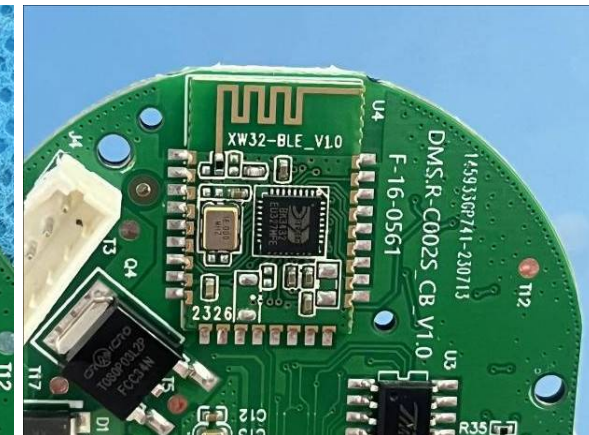
RF Module
