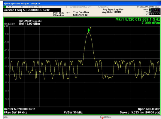
NT/NV_Antenna 0 IEEE 802.11n_Channel 64_20MHz
