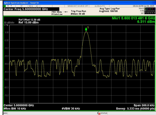
NT/NV_Antenna 0 IEEE 802.11n_Channel 120_20MHz
