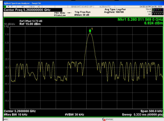
NT/NV_Antenna 0 IEEE 802.11n_Channel 52_20MHz
