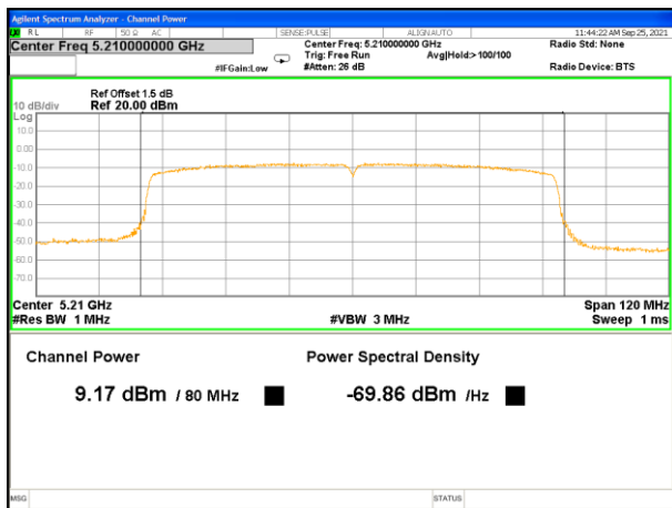
5210MHz_AV_Ant B
