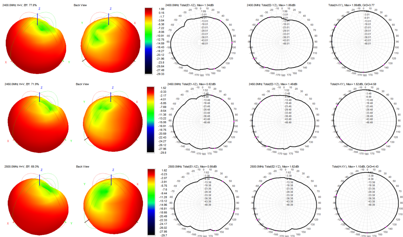
天线场型图
