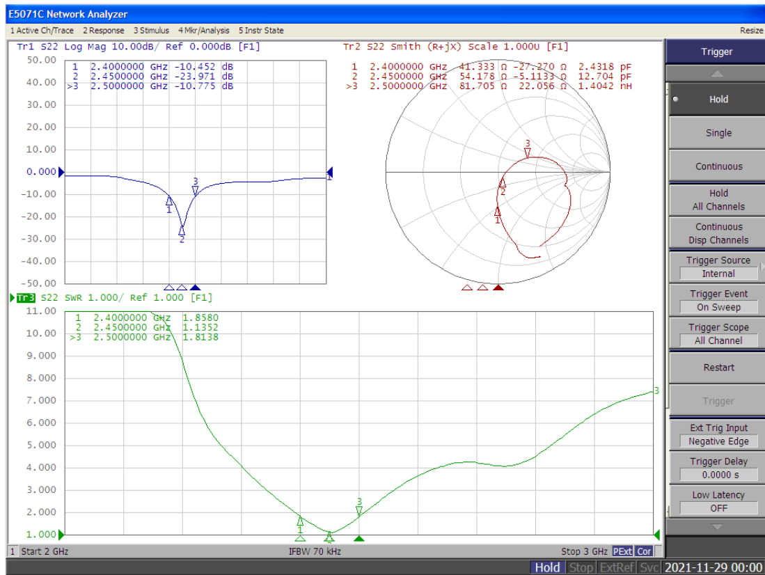
天线 S 参数
