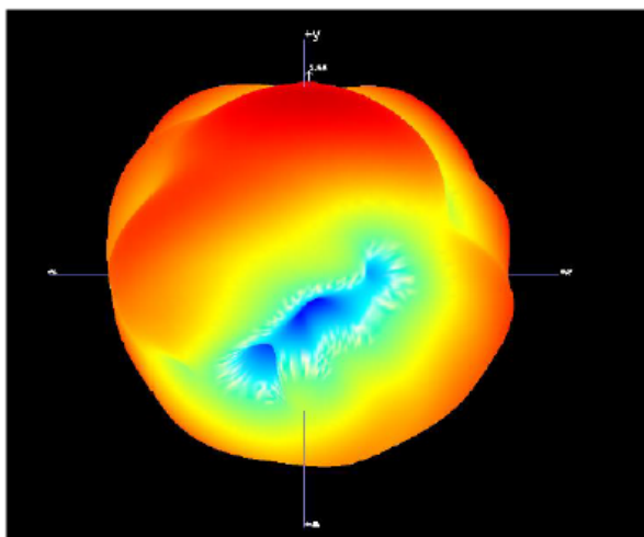
2400Mhz
