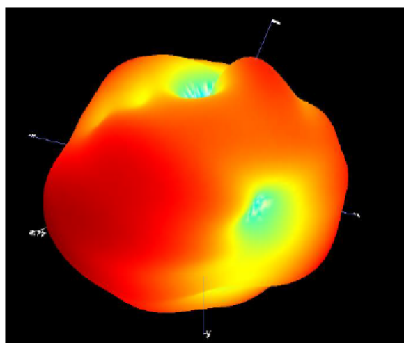
2483Mhz
