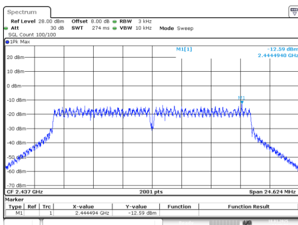
802.11g_2437MHz
