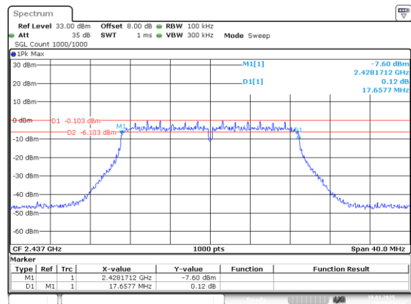
802.11n20_2437MHz
