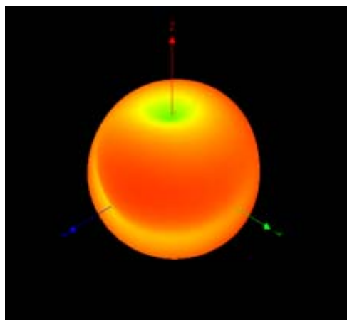
2500MHz
