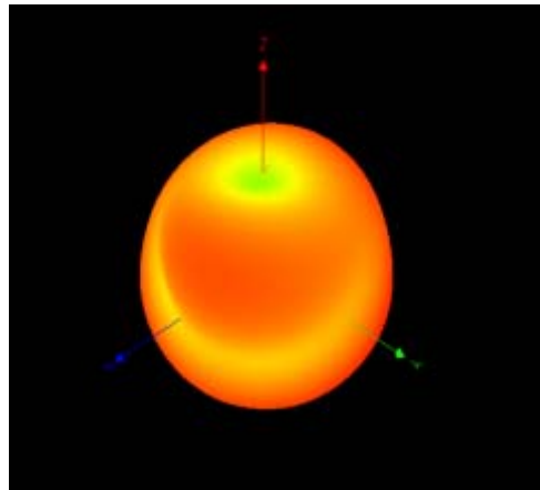
2400MHz
