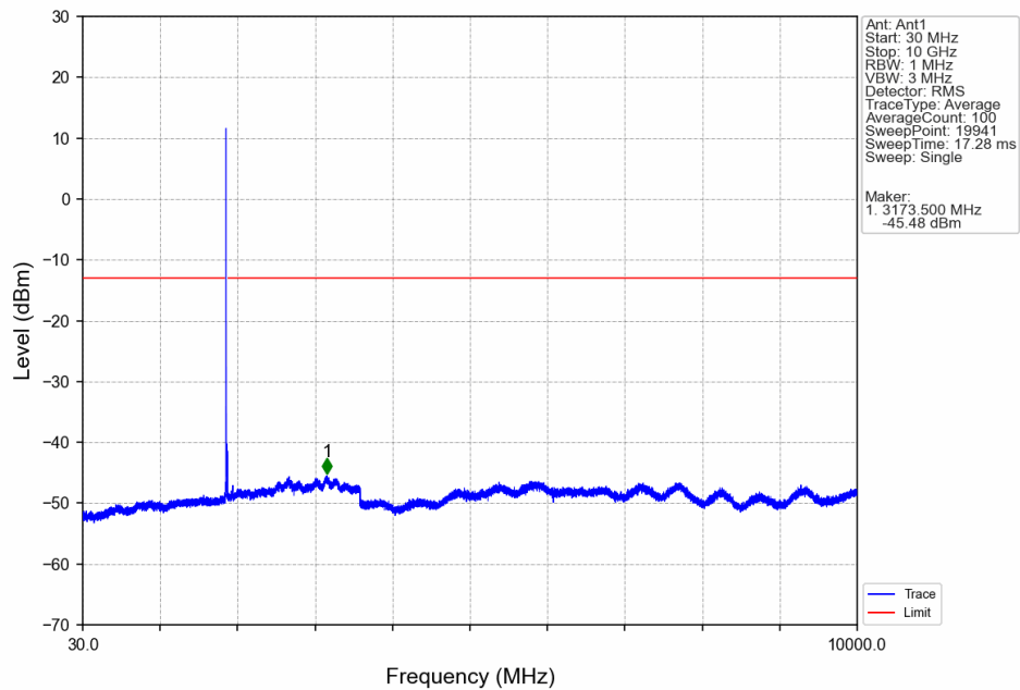
Band2_10MHz_16QAM_MCH_1880MHz_RB_1_0_NTV
