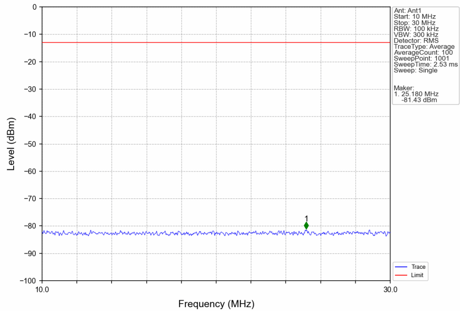
Band2_10MHz_16QAM_MCH_1880MHz_RB_1_0_NTV
