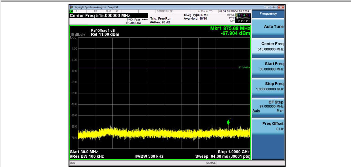
2.4G-Ant1-2405-30~1000-PASS
