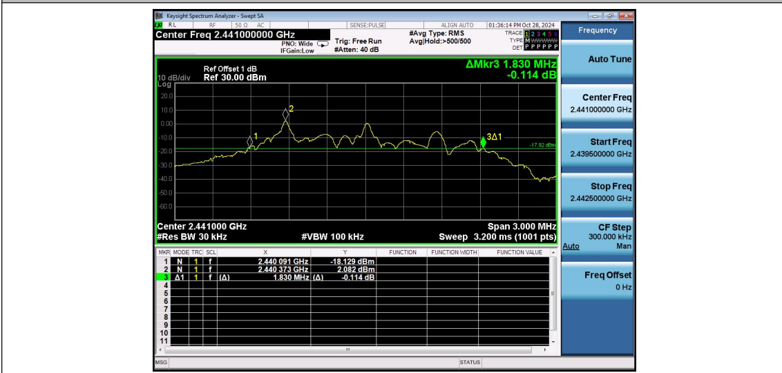
2.4G-Ant1-2441
