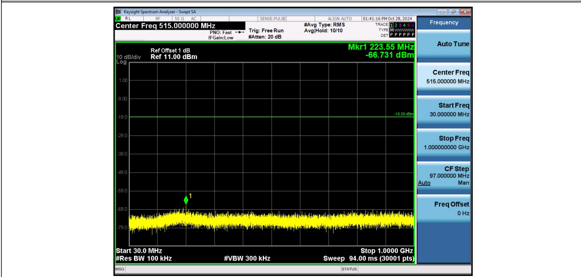
2.4G-Ant1-2475-30~1000-PASS
