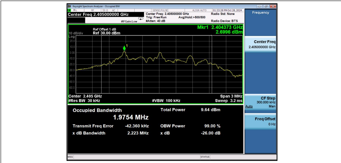
2.4G-Ant1-2405
