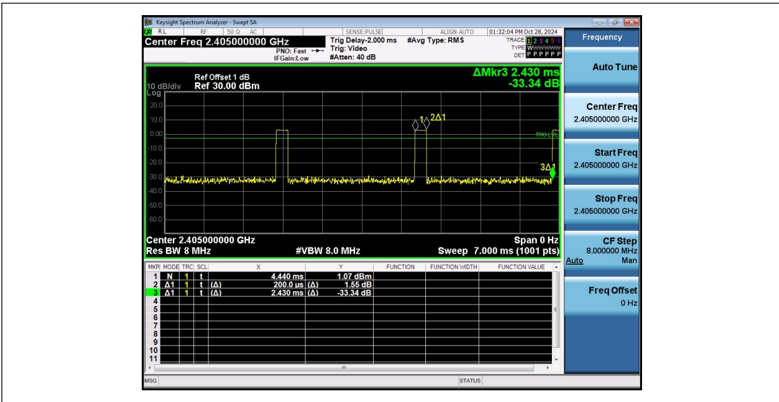
NTNV-2.4G-Ant1-2405
