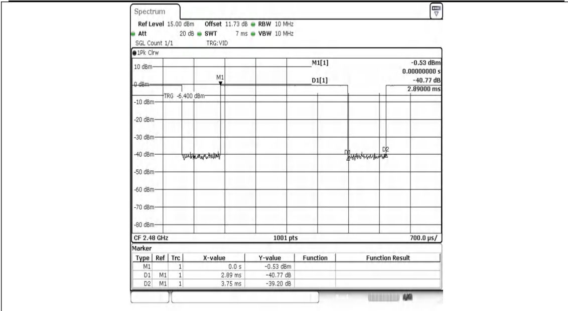
NTNV-DH5-Ant1-2480
