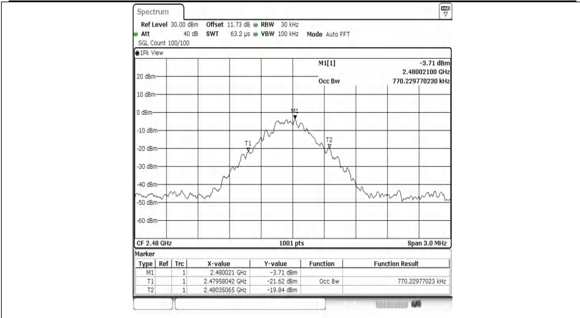
DH5-Ant1-2480
