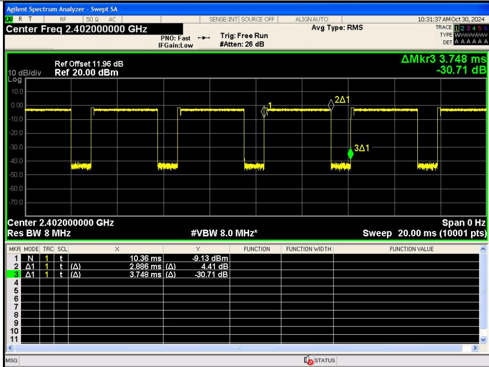
\pi/4 DQPSK(2-DH5)_Channel 0
