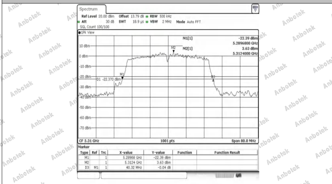
11N40SISO-Ant1-5310
