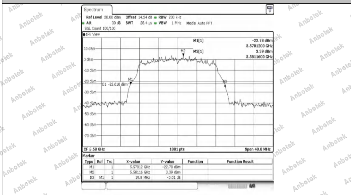
11A-Ant1-5580
