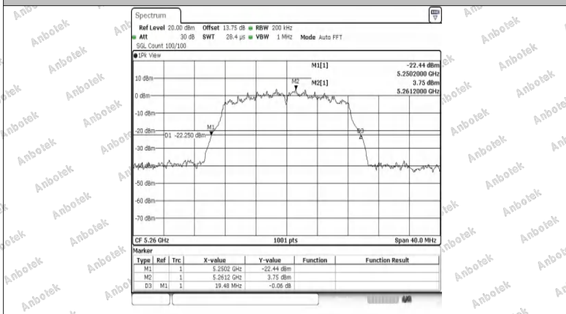
11A-Ant1-5260
