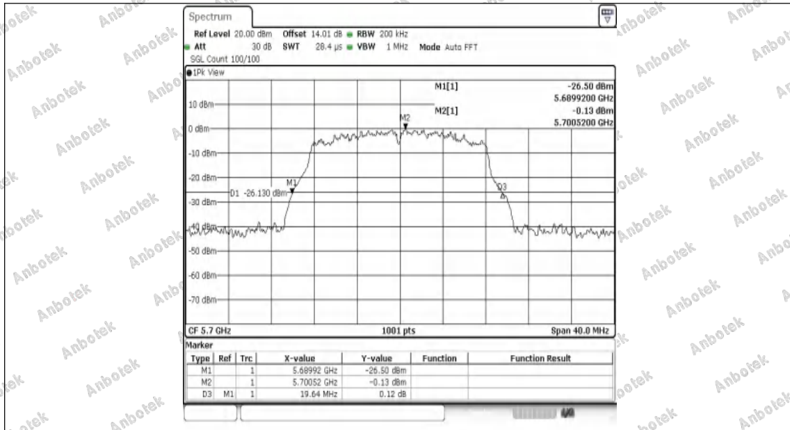
11A-Ant1-5700
