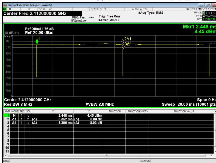
802.11b
