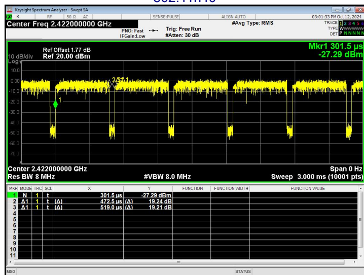
802.11n40
