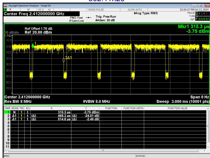
802.11n20
