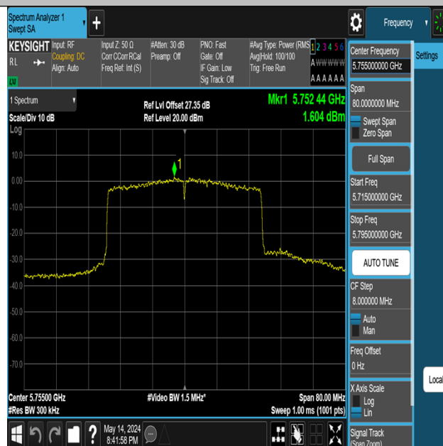
11AX40MIMO-Ant3-5755-PASS
