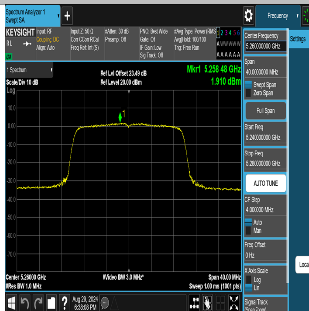
11AX20MIMO-Ant1-5260-PASS
