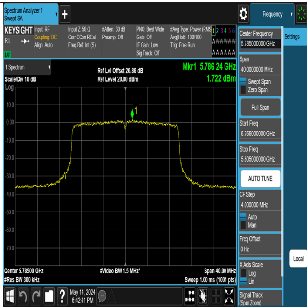
11AX20MIMO-Ant1-5785-PASS
