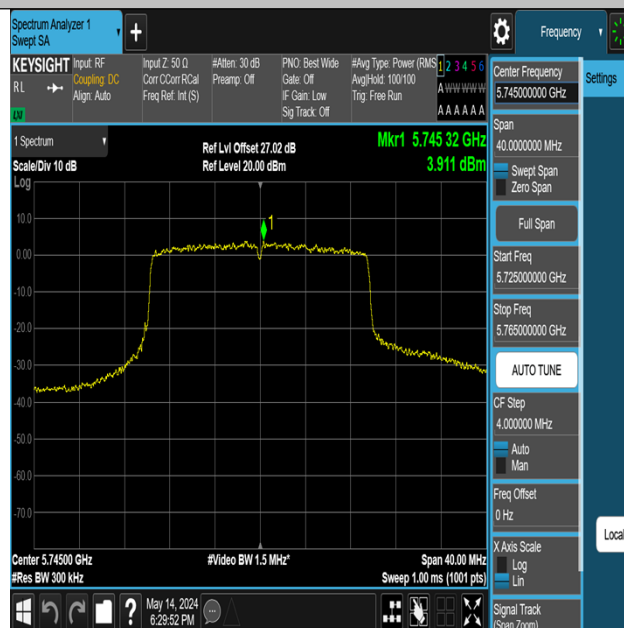
11AX20MIMO-Ant3-5745-PASS
