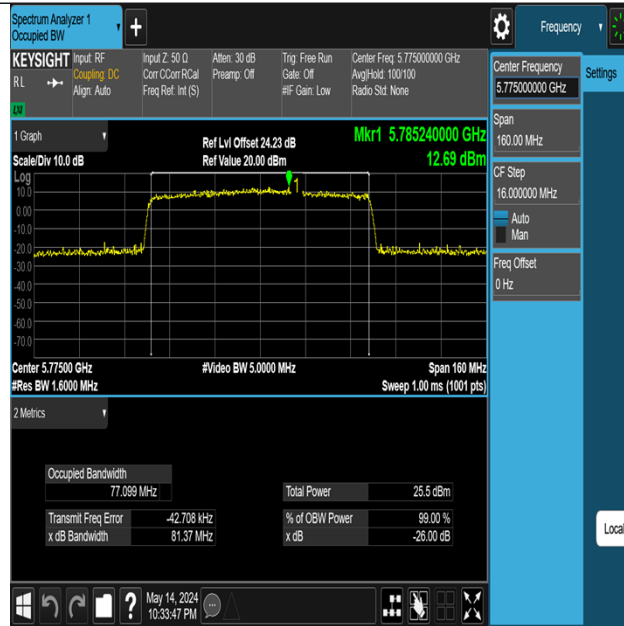
11AX80MIMO-Ant3-5775
