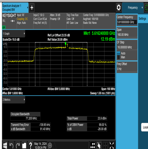
11AX80MIMO-Ant1-5610
