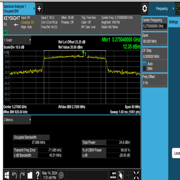
11AX40MIMO-Ant3-5270
