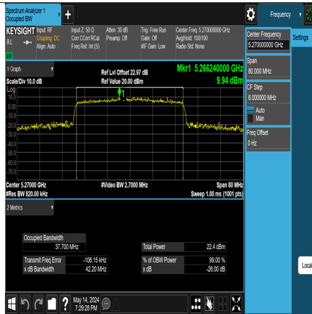
11AX40MIMO-Ant2-5270
