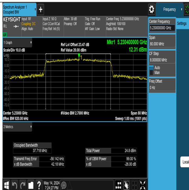
11AX40MIMO-Ant3-5230
