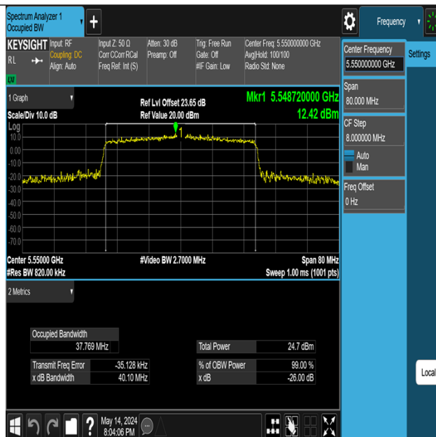
11AX40MIMO-Ant3-5550
