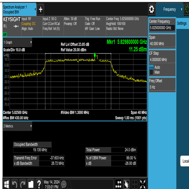
11AX20MIMO-Ant3-5825
