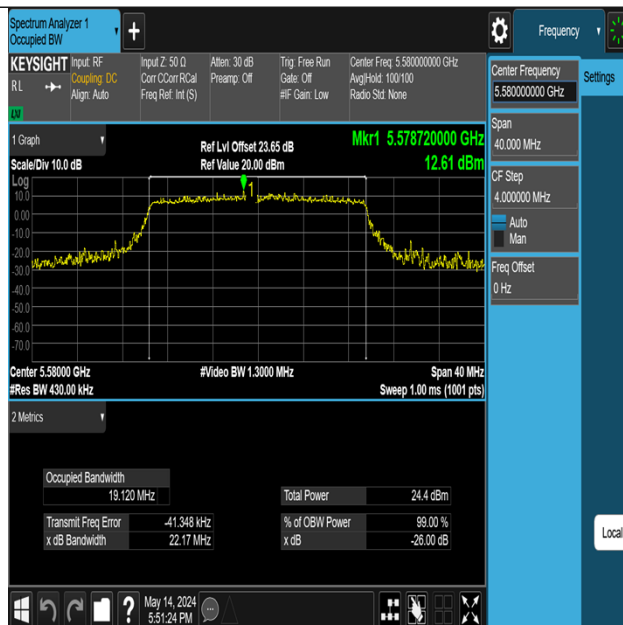
11AX20MIMO-Ant3-5580
