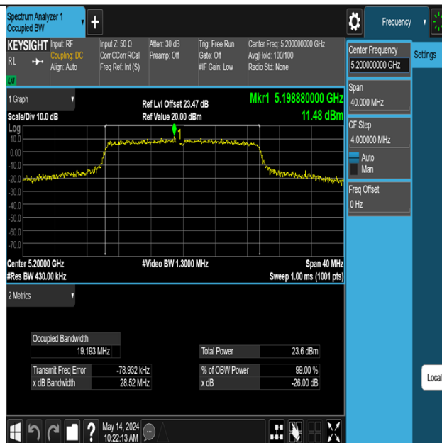
11AX20MIMO-Ant3-5200
