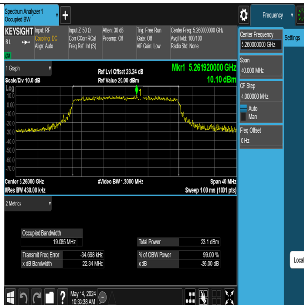
11AX20MIMO-Ant1-5260
