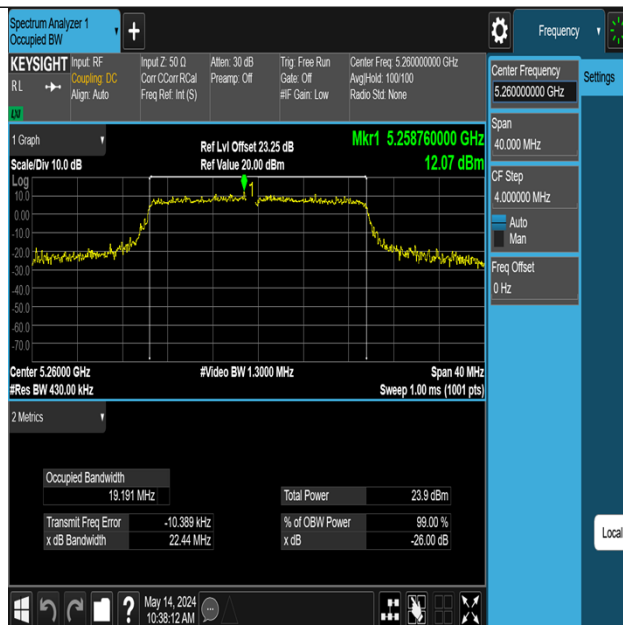
11AX20MIMO-Ant3-5260
