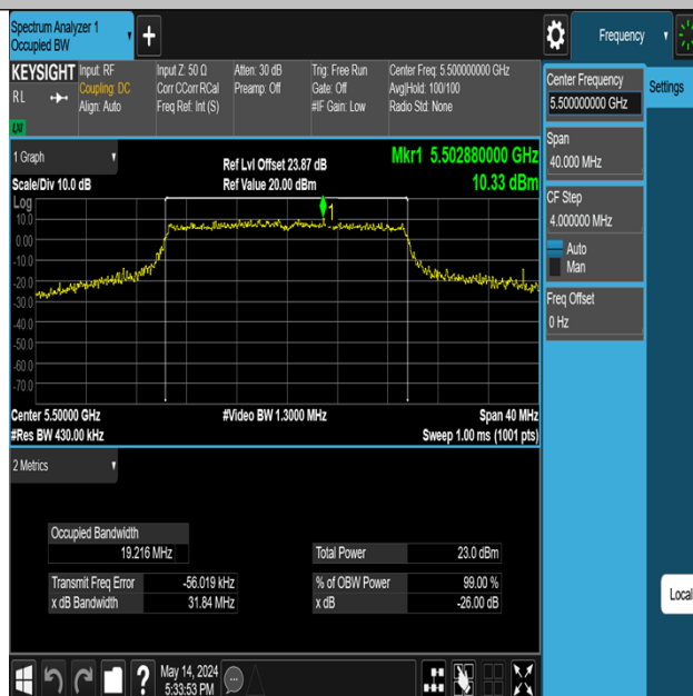
11AX20MIMO-Ant1-5500
