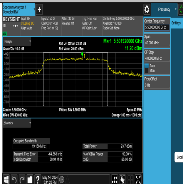
11AX20MIMO-Ant3-5500
