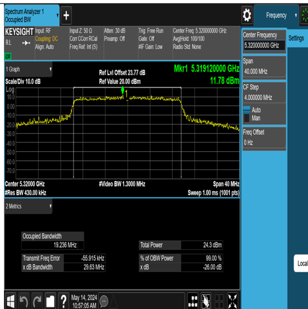
11AX20MIMO-Ant3-5320
