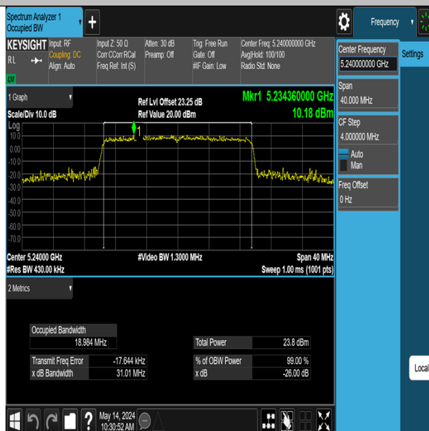
11AX20MIMO-Ant3-5240
