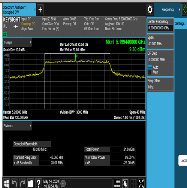
11AX20MIMO-Ant2-5200
