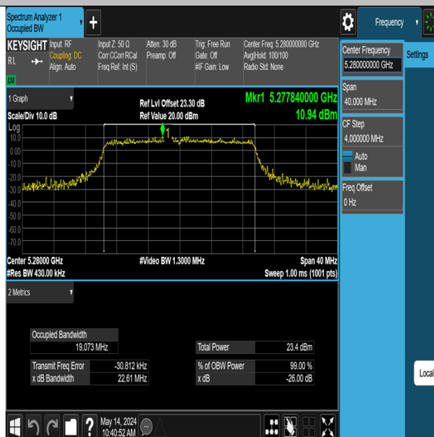
11AX20MIMO-Ant1-5280
