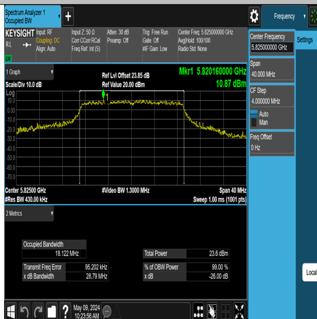
11N20MIMO-Ant3-5825
