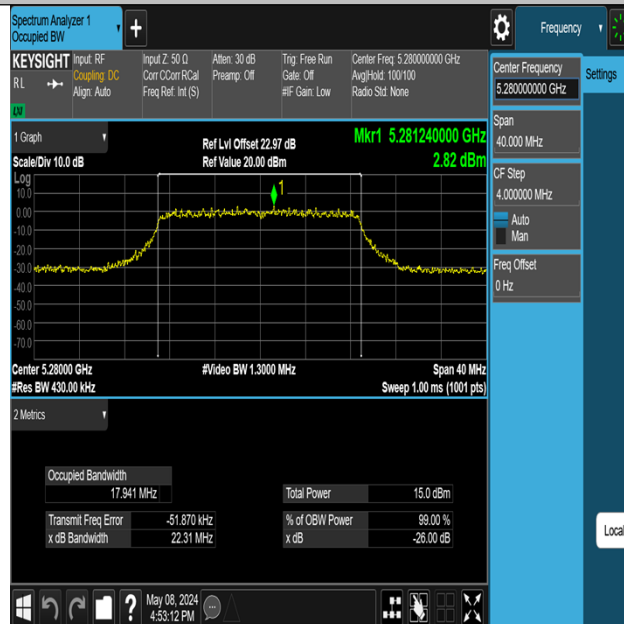
11N20MIMO-Ant2-5280
