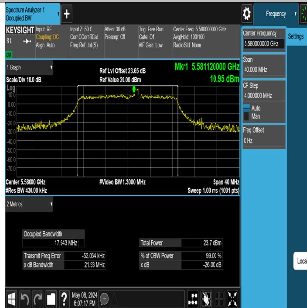
11N20MIMO-Ant3-5580
