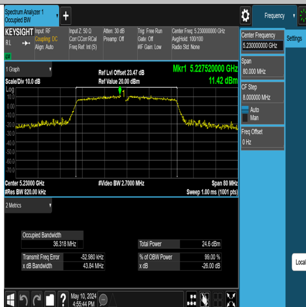
11N40MIMO-Ant3-5230
