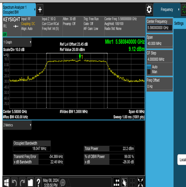
11N20MIMO-Ant1-5580
