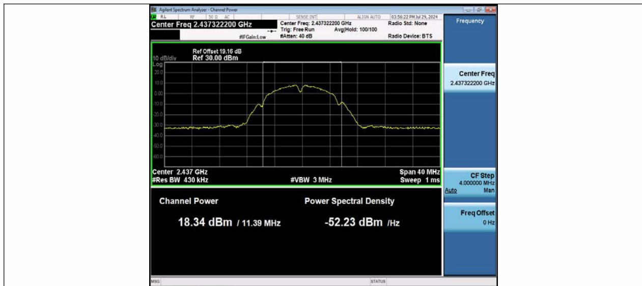
11B_Ant2_2437
