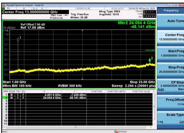
1G-25G
