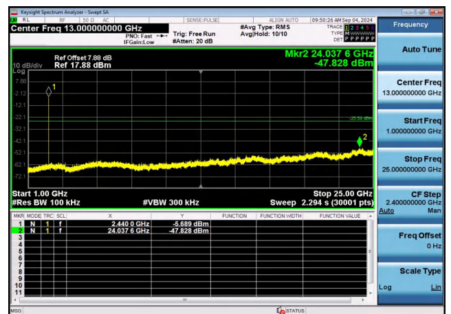
1G-25G
