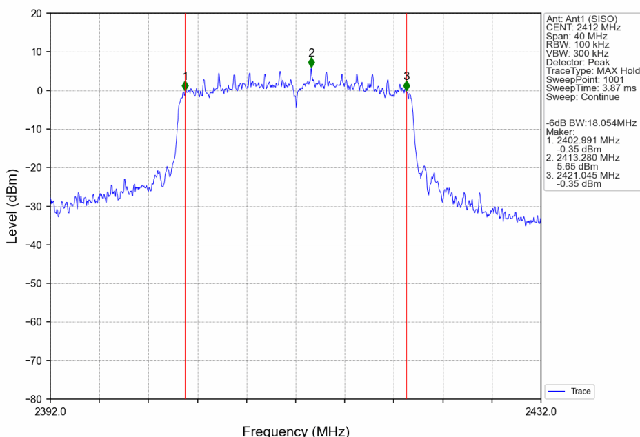
802.11ax(HEW20)_LCH_2412MHz_SU_Ant1 (SISO)_NTNV
