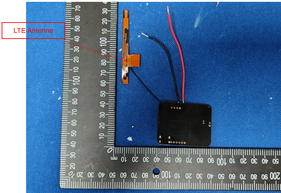
EUT Photo
