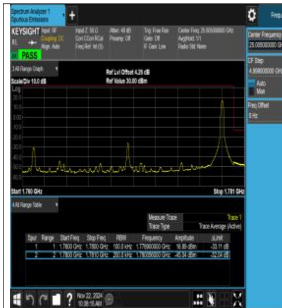
Band66_20MHz_QPSK_132572_1RB#99
