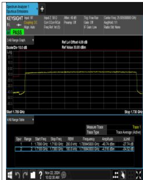
Band66_20MHz_QPSK_132072_100RB#0
