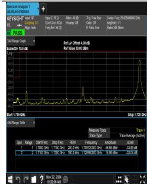
Band66_20MHz_QPSK_132072_1RB#99
