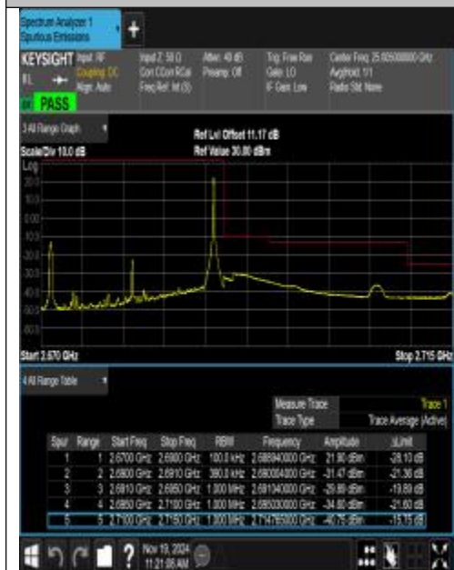
Band41_20MHz_QPSK_41490_1RB#99
