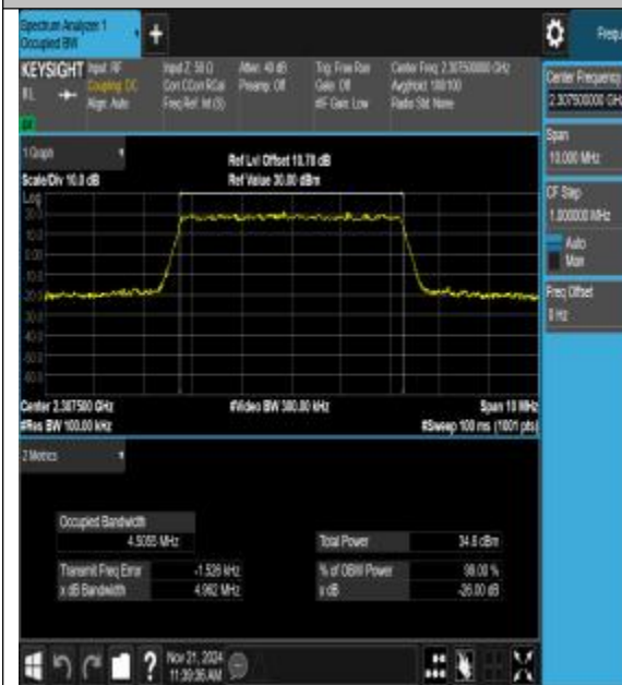
40(2305-2320)-5MHz-QPSK-38725-25RB#0-PAS
