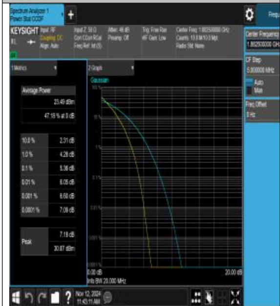
Band25-20MHz-QPSK-26365-100RB#0-PASS
