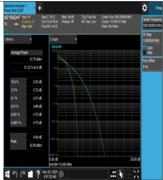
26(824-849)-10MHz-16QAM-26915-1RB#0-PASS
