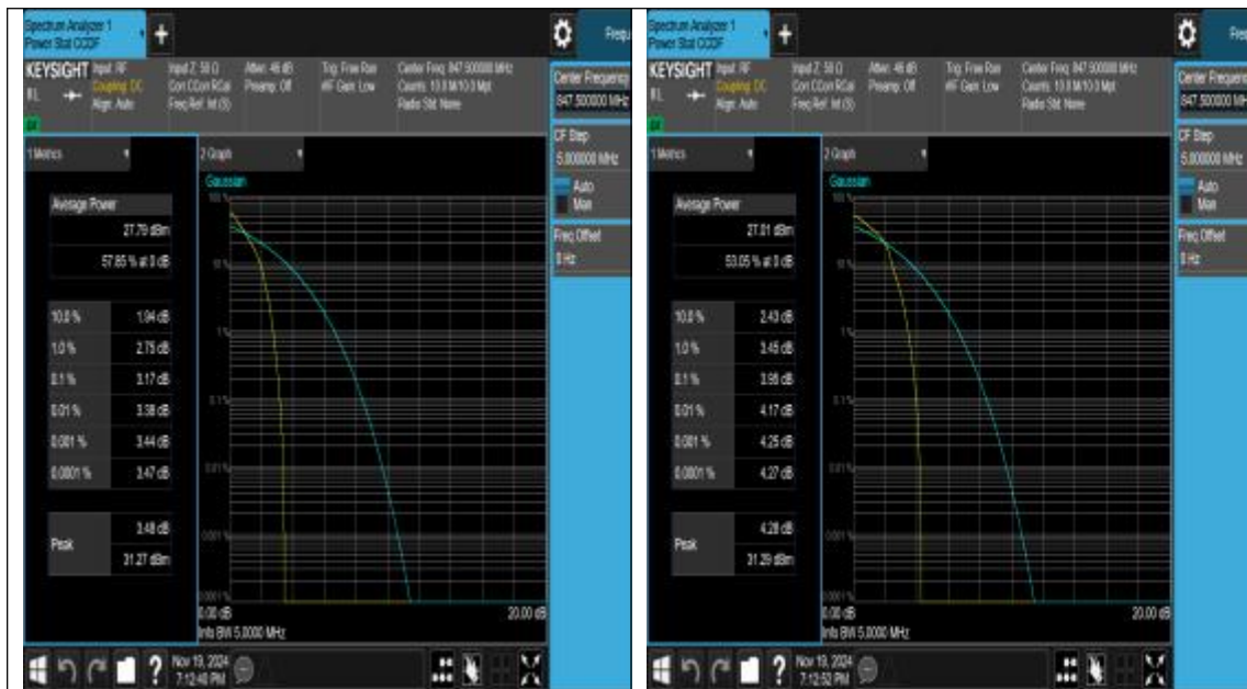
26(824-849)-3MHz-QPSK-27025-1RB#0-PASS
