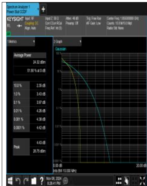
Band2-10MHz-QPSK-18650-1RB#0-PASS
