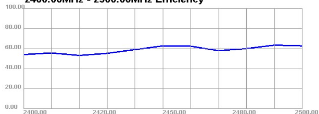
2400.00MHz - 2500.00MHz Efficiency
