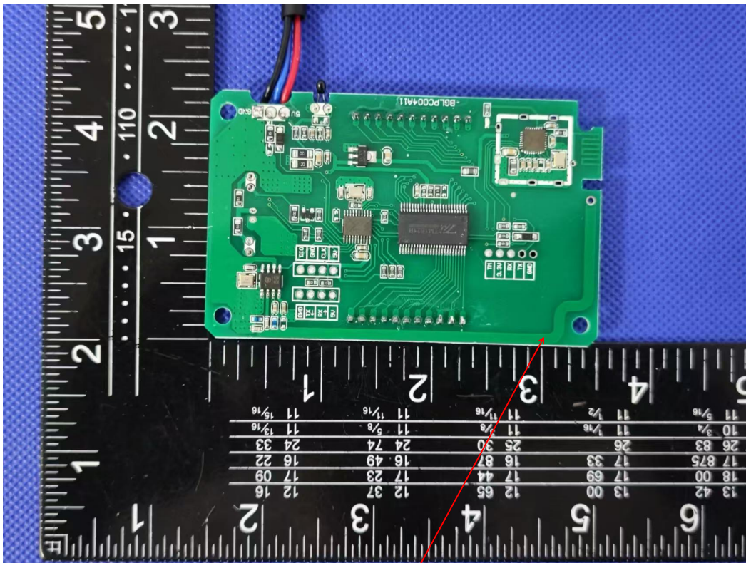
433.92 RX ANT
