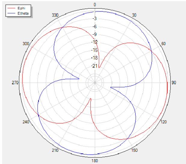
Theta=0 freq=2500MHz
