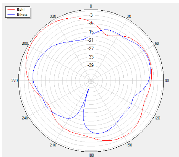
Theta=90 freq=2400MHz
