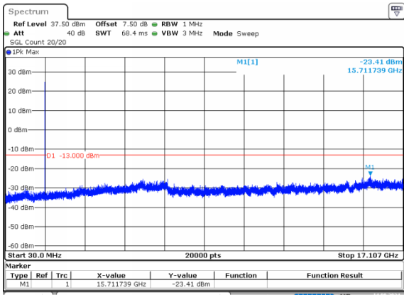
1.4MHz_Low_QPSK_1@0
