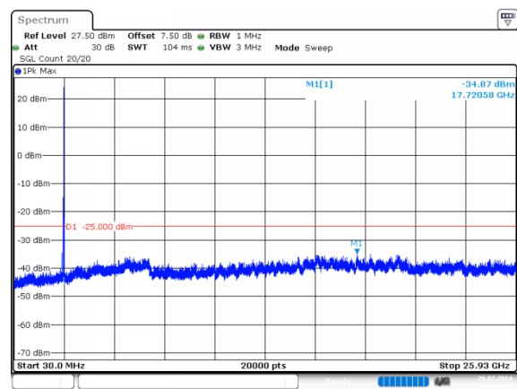
20MHz_Middle_QPSK_1@0
