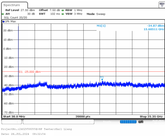
10MHz_Low_QPSK_1@0
