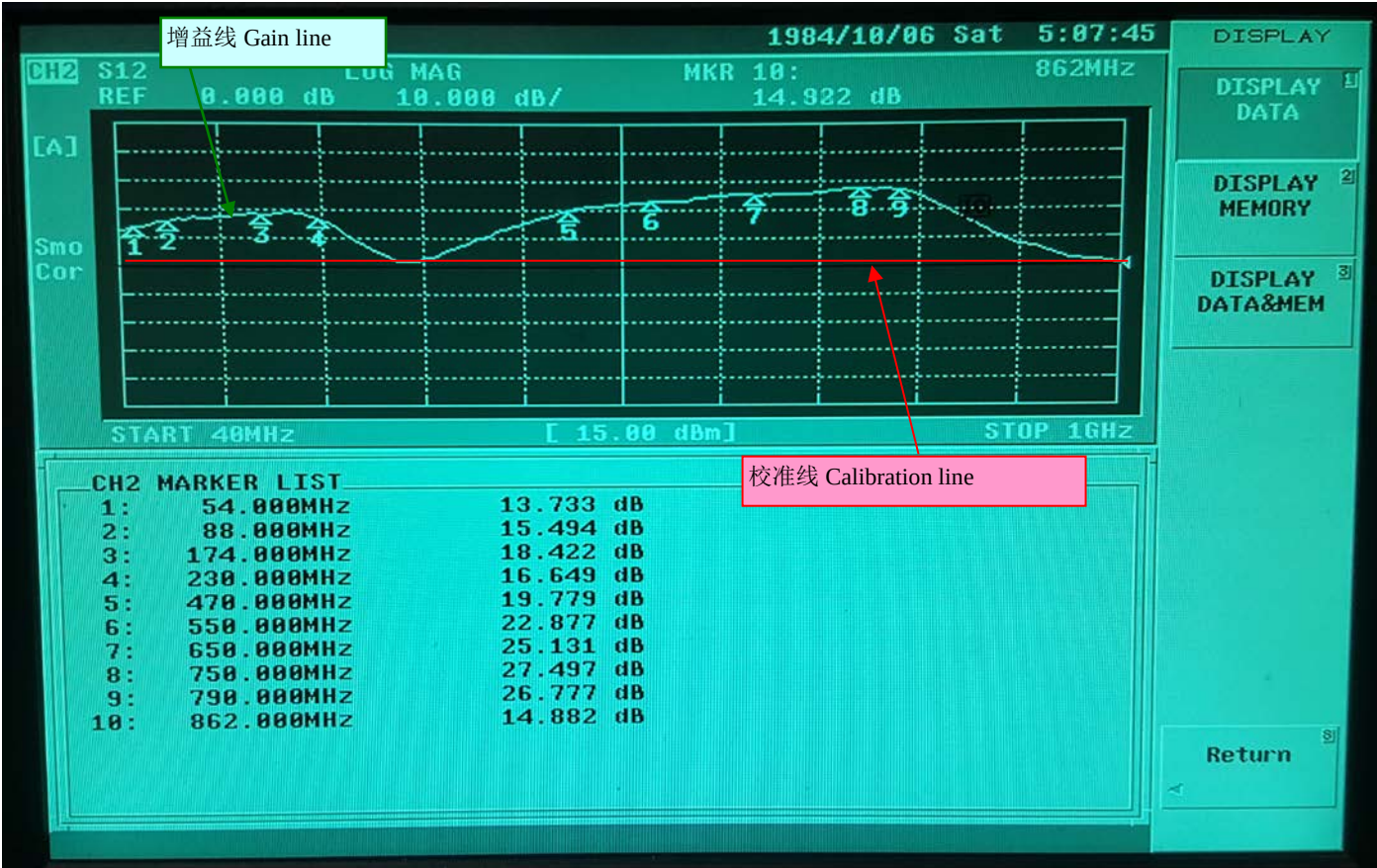
增益测试图 Gain test chart
