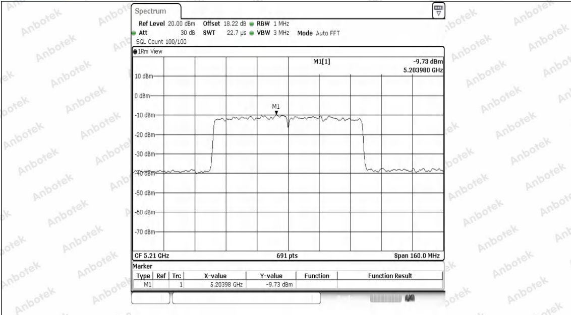
11AC80SISO-Ant1-5210-PASS
