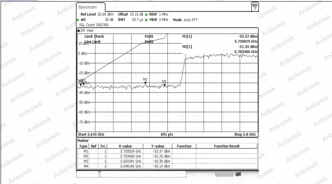
11AC80SISO-Ant1-5775-PASS
