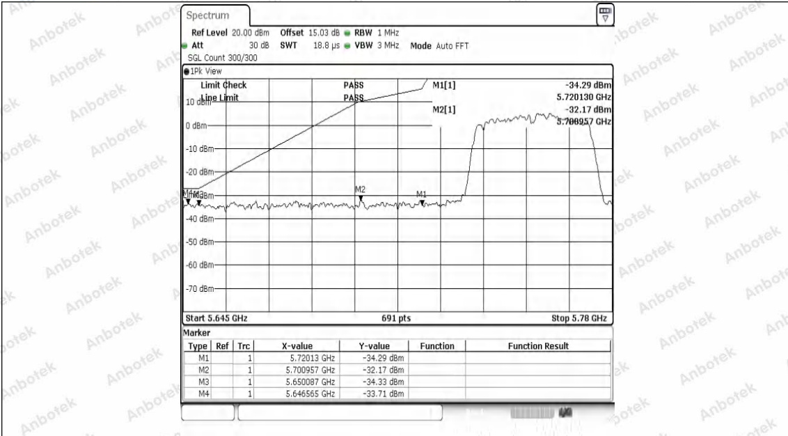
11N40ISO-Ant1-5755-PASS
