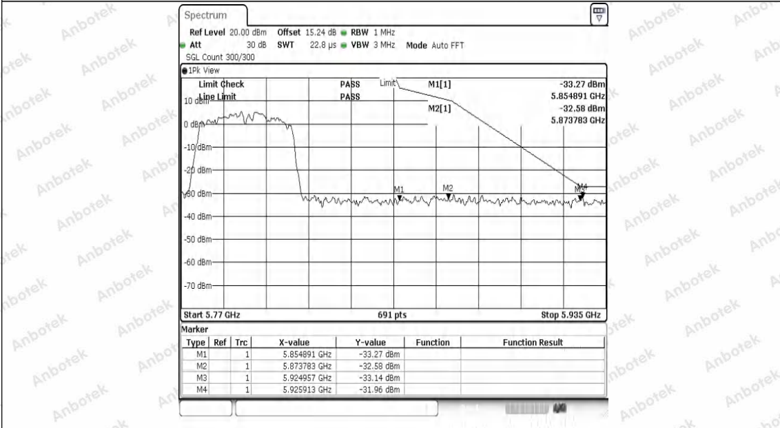
11N40ISO-Ant1-5795-PASS
