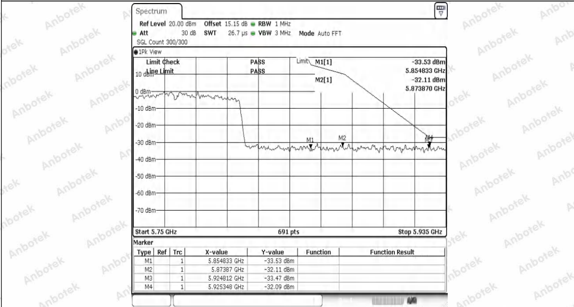
11AC80SISO-Ant1-5775-PASS
