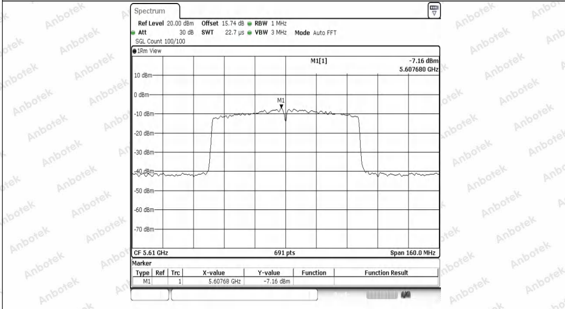
11AC80SISO-Ant1-5610-PASS
