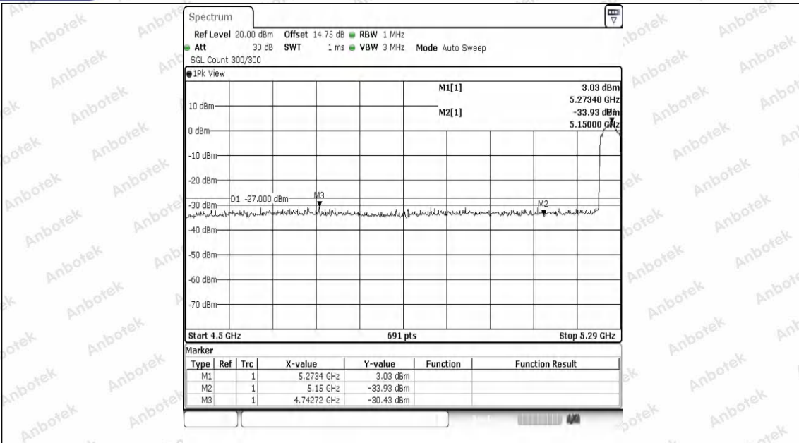
11N40SISO-Ant1-5270-PASS
