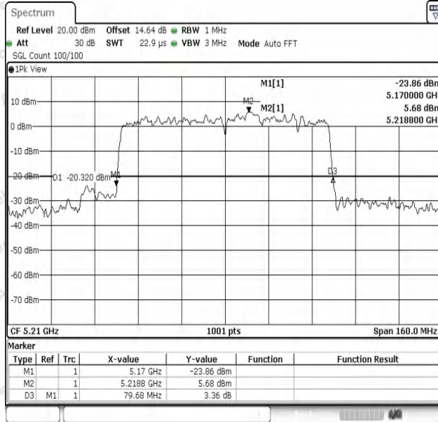
11AC80SISO-Ant1-5210
