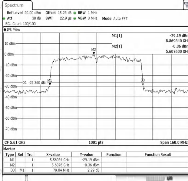
11AC80SISO-Ant1-5610
