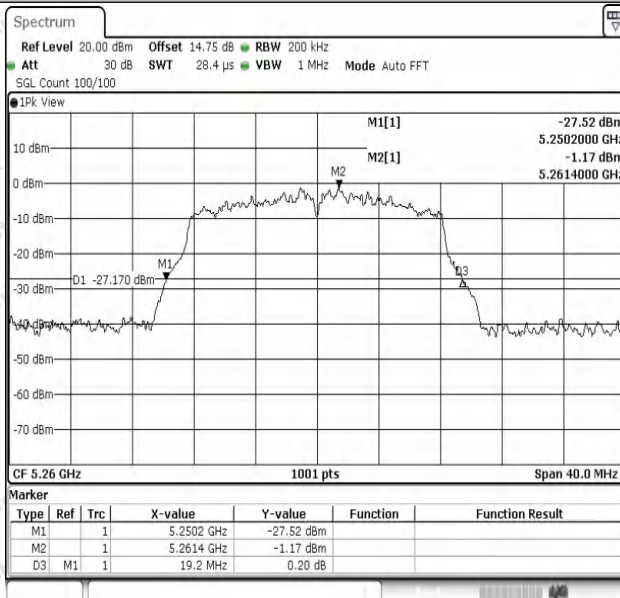
11A-Ant1-5260
