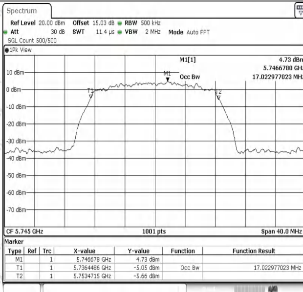
11A-Ant1-5745
