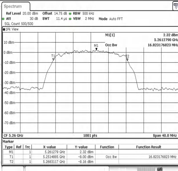
11A-Ant1-5260
