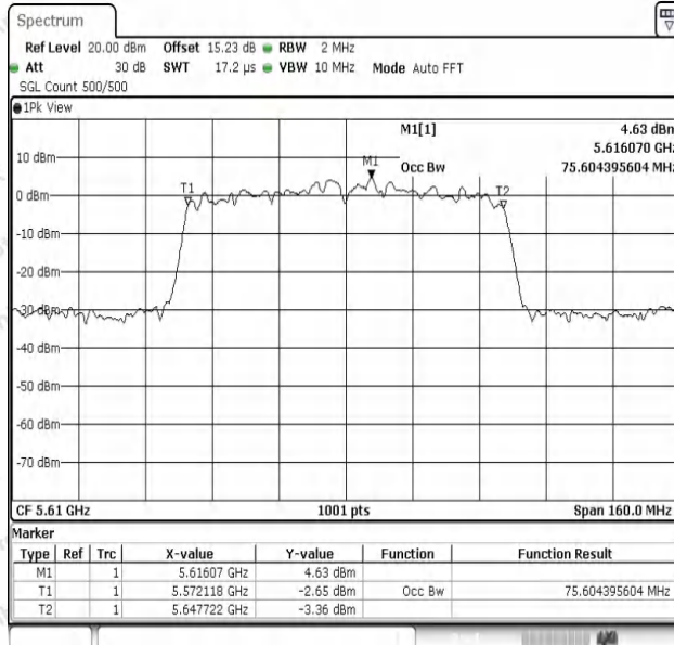
11AC80SISO-Ant1-5610
