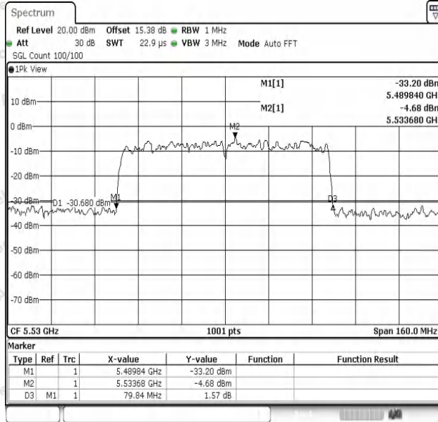
11AC80SISO-Ant1-5530
