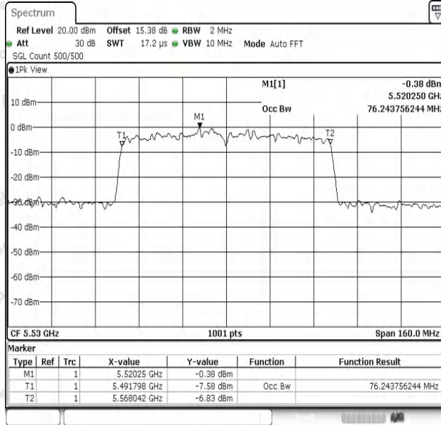
11AC80SISO-Ant1-5530
