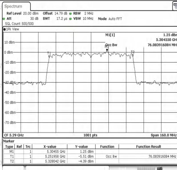
11AC80SISO-Ant1-5290
