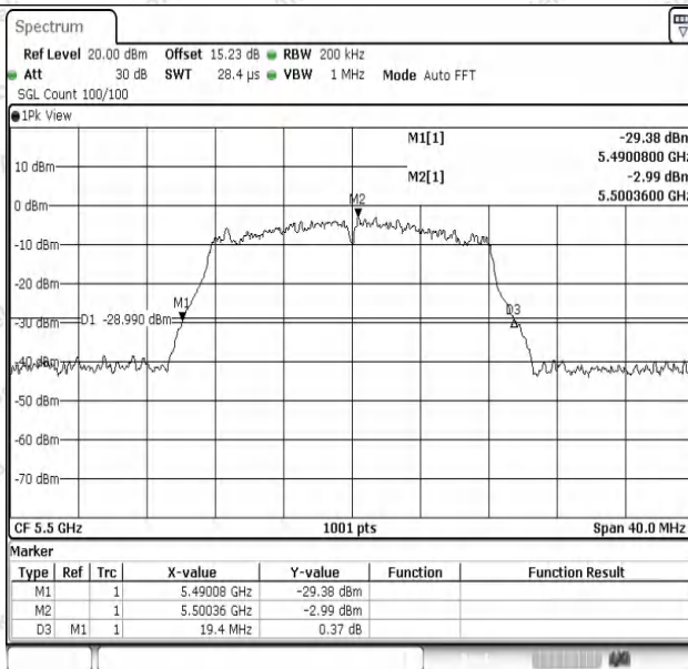
11A-Ant1-5500
