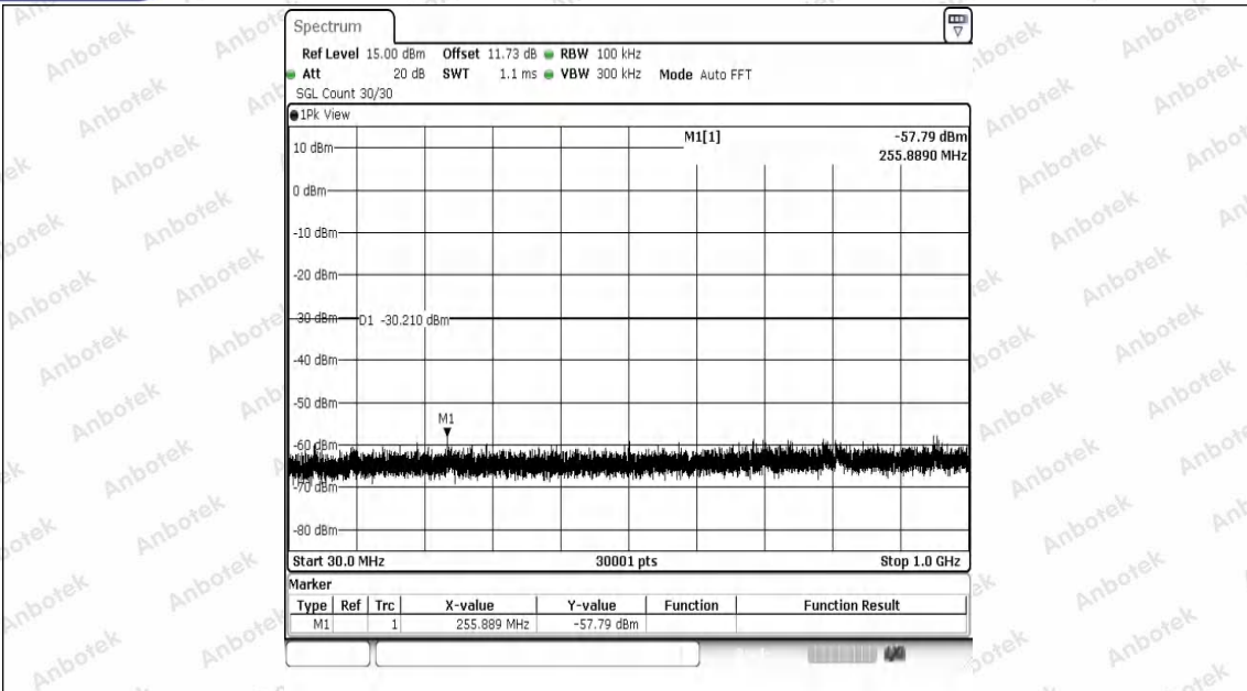
11G-Ant1-2462-30~1000-PASS
