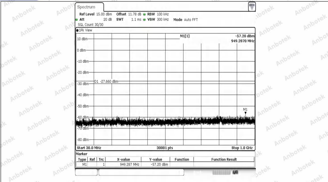
11G-Ant1-2412-30~1000-PASS
