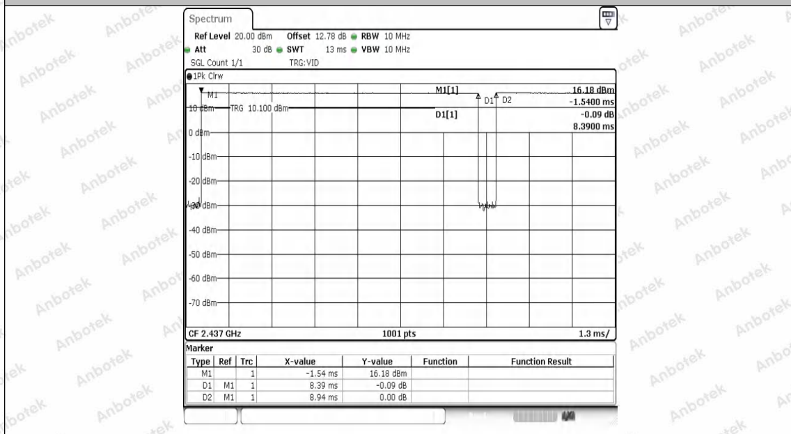
NTVN-11B-Ant1-2437
