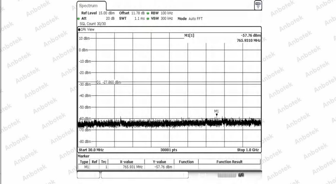
11G-Ant1-2437-30~1000-PASS
