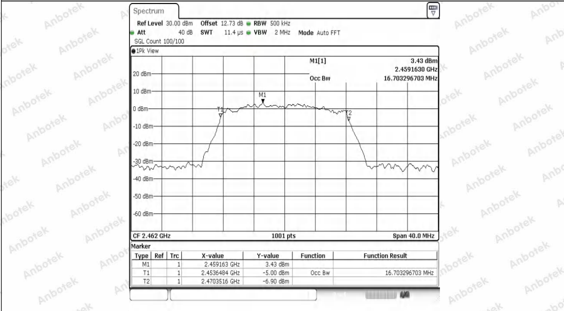
11G-Ant1-2462
